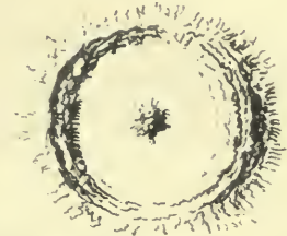
TYCHO. 50 Miles Diam r
